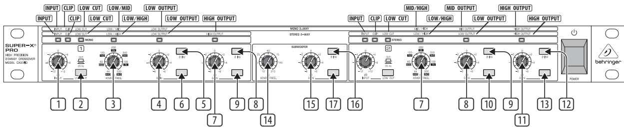
図 2.3: モノラル 3 ウェイ / 独立サブウーファー信号モードで使用される、SUPER-X PRO フロントパネル上のアクティブコントローラー・スイッチ類
