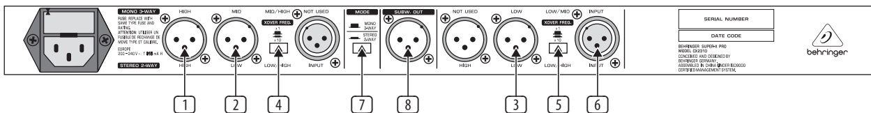
図 2.4: モノラル 3 ウェイ / 独立サブウーファー信号モードで使用される、SUPER-X PRO 後部のアクティブコントローラー類とコネクタ
