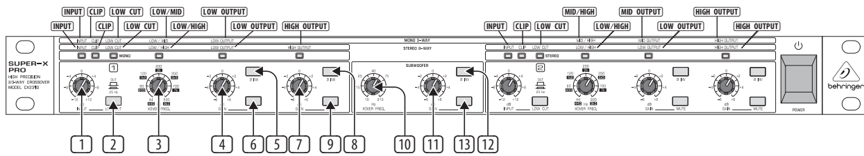
図 2.1: ステレオ 2 ウェイ / 独立サブウーファー信号モードで使用される、SUPER-X PRO フロントパネルのアクティブ・コントローラー / スイッチ類
