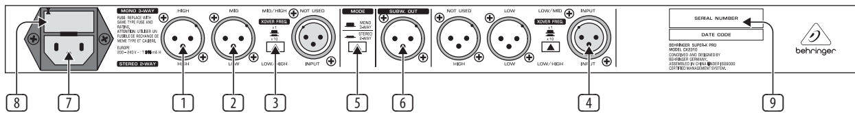
図 2.2: ステレオ 2 ウェイ・モード / 独立サブウーファー信号モードで使用される SUPER-X PRO 後部のアクティブ・コントローラー類とコネクター
